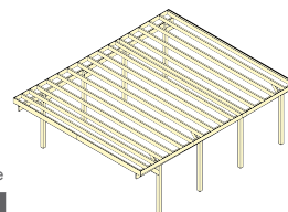
Coffrage en bois, bande bitumineuse
